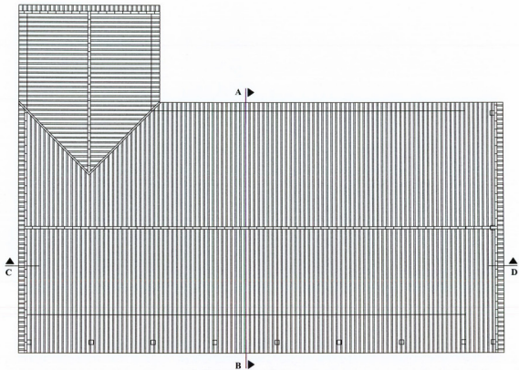
PLANTA DE COBERTURA
