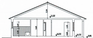
CORTE A - B
