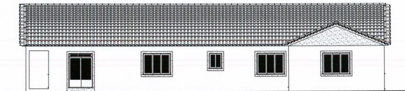
ALÇADO POSTERIOR
