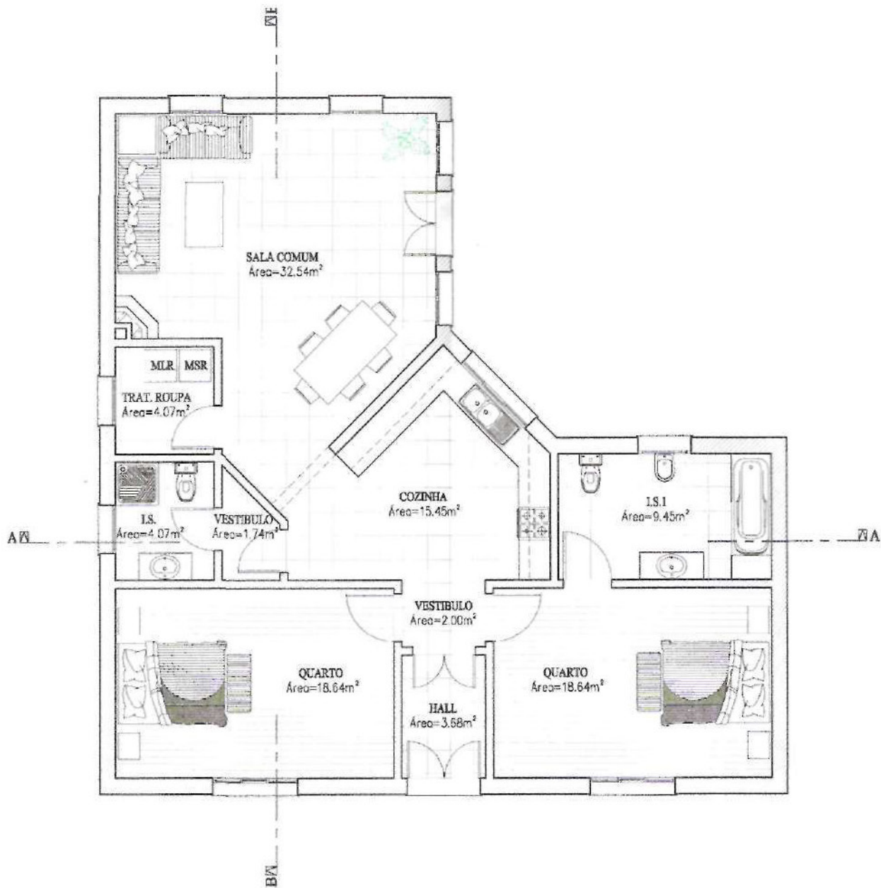
PLANTA DO PISO 0
