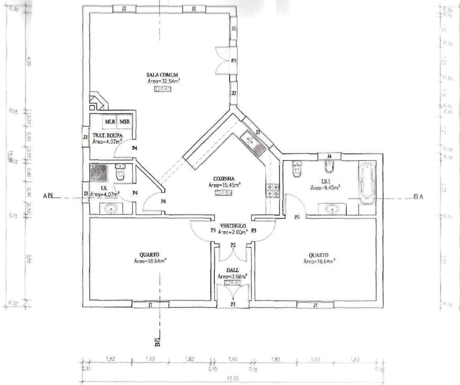
PLANTA DO PISO 0
